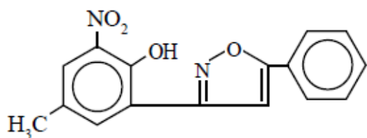
Ligand-I
