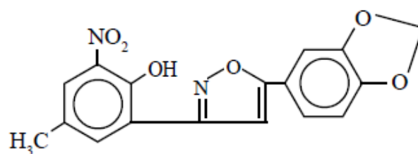
Ligand-IV
