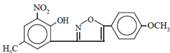
Ligand-II
